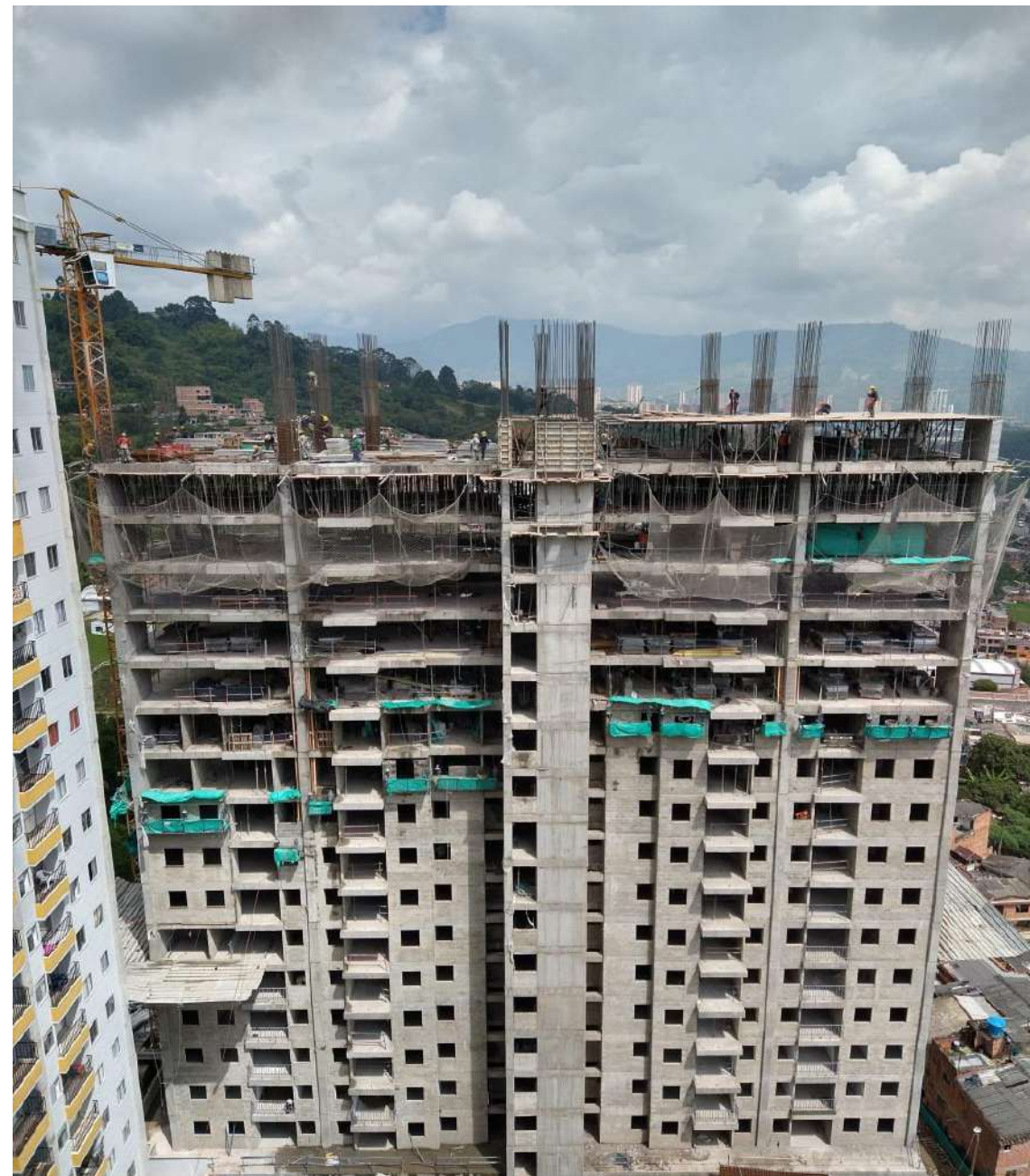
Estructura torre 3 – armado losa p17 y losa p1 plataforma central
