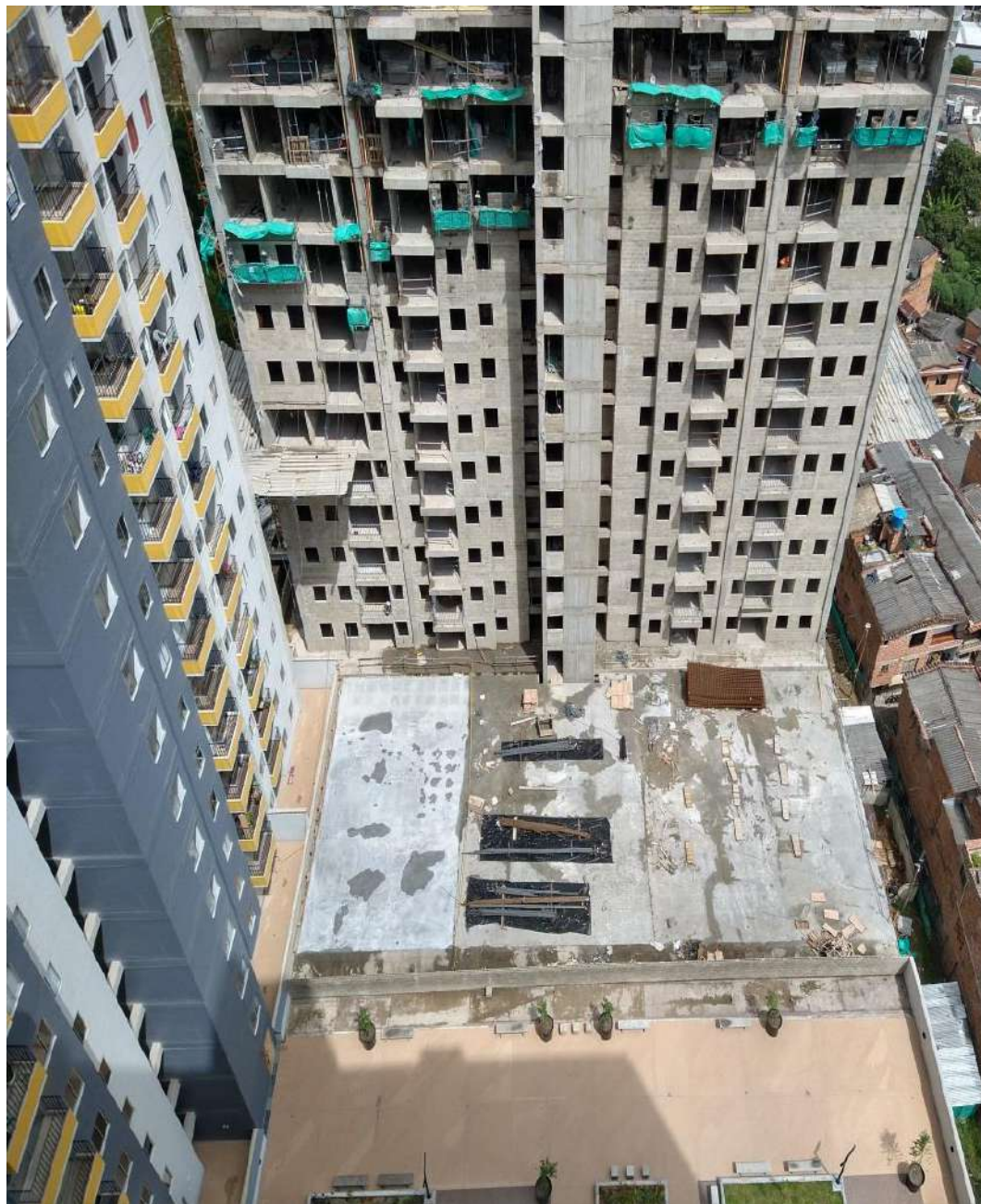
Estructura torre 3 – armado losa p17 y losa p1 plataforma central
