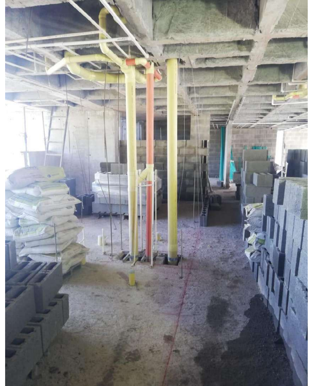
Mampostería interna piso 12 torre 3 y de fachadas torre 3 piso 10
